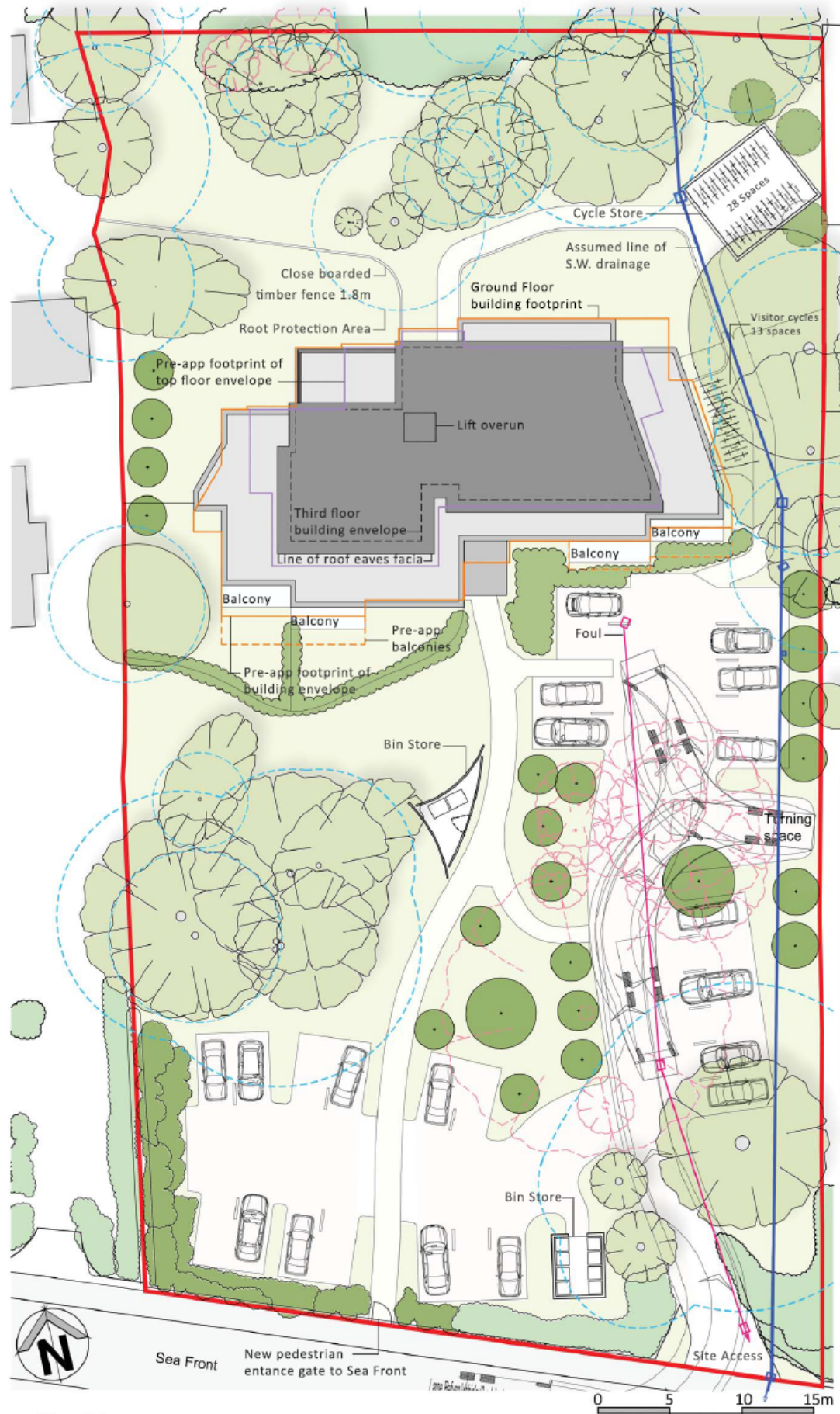
Site Plan 1:250@A3
